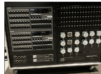
移動式分岐盤 FK x 5 系統(メスx1, オスx2) +Y009/Y010
